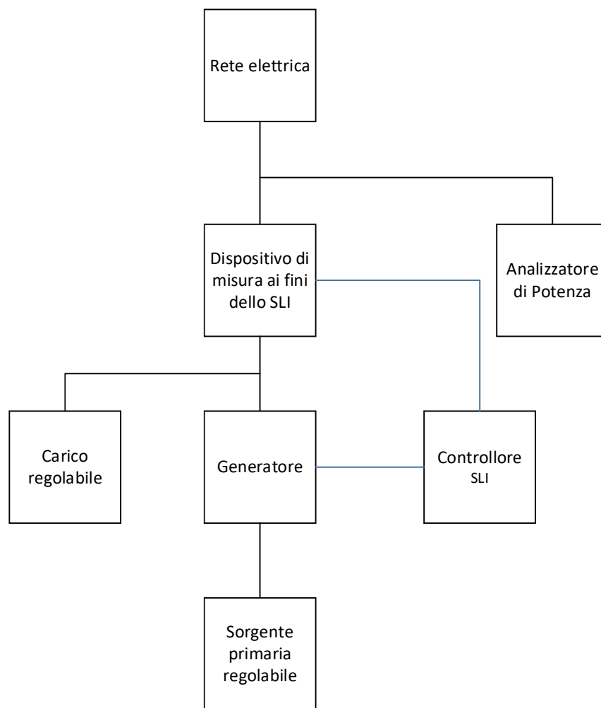
Figura L.5- Schema a blocchi delle prove
